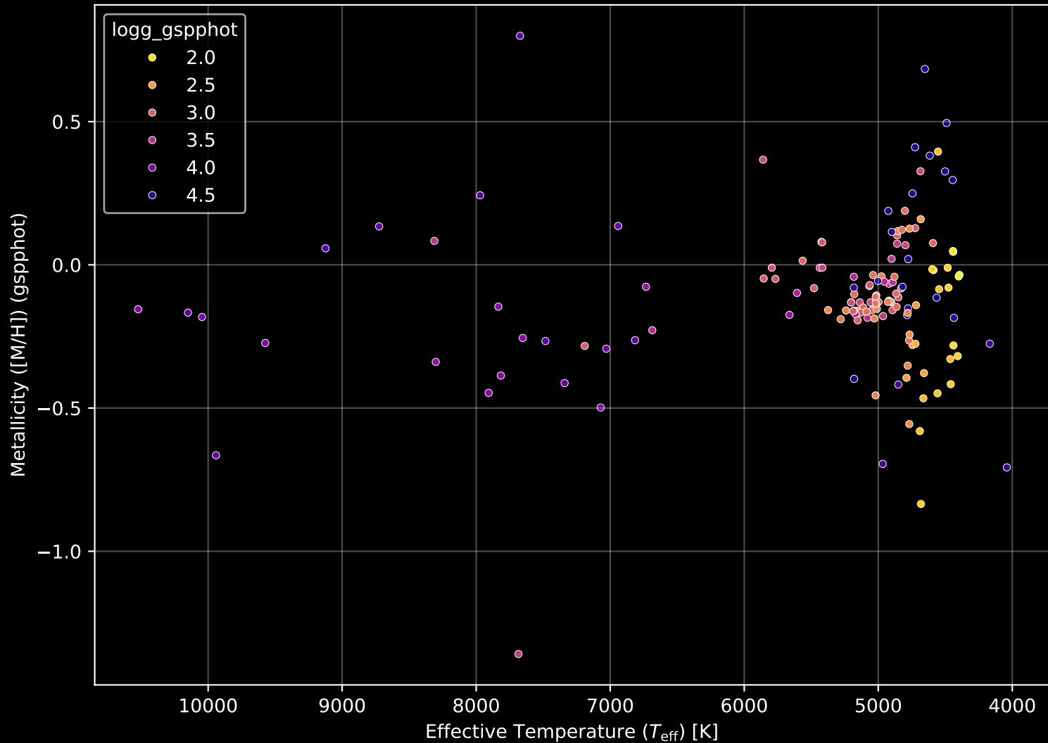
APOGEE DR17 Field: [150+16] Stellar Population Parameters (n= 147)
